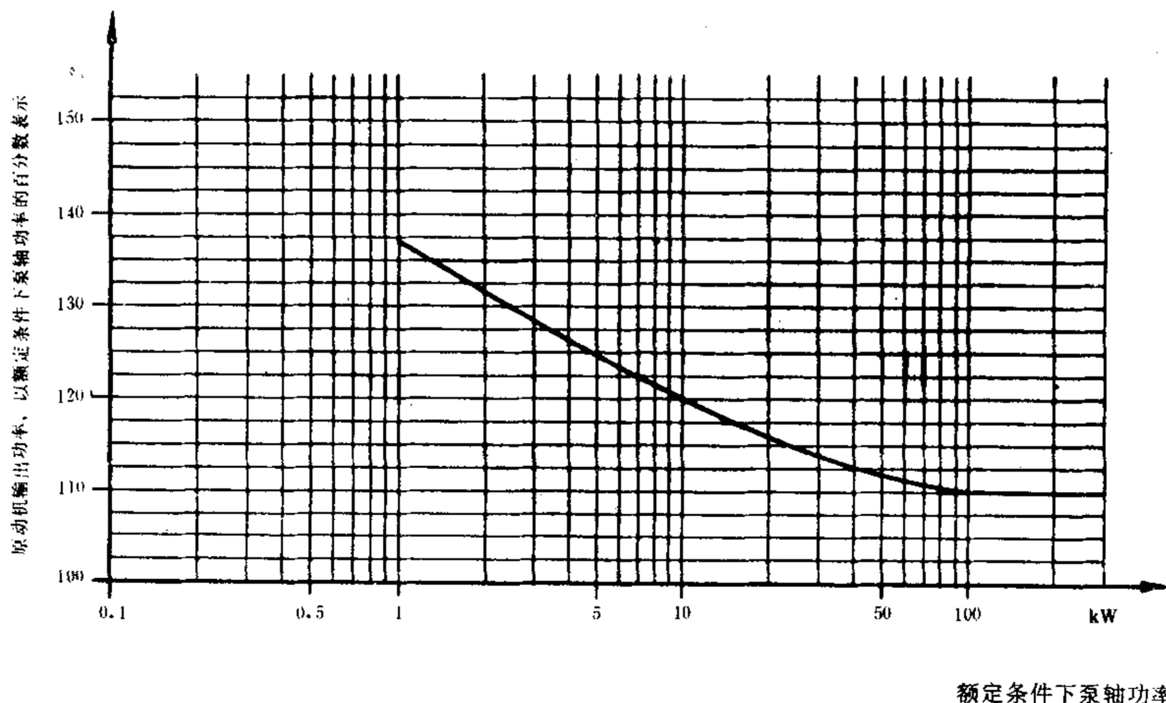
图 2 以额定条件下泵轴功率的百分数表示的原动机输出功率
