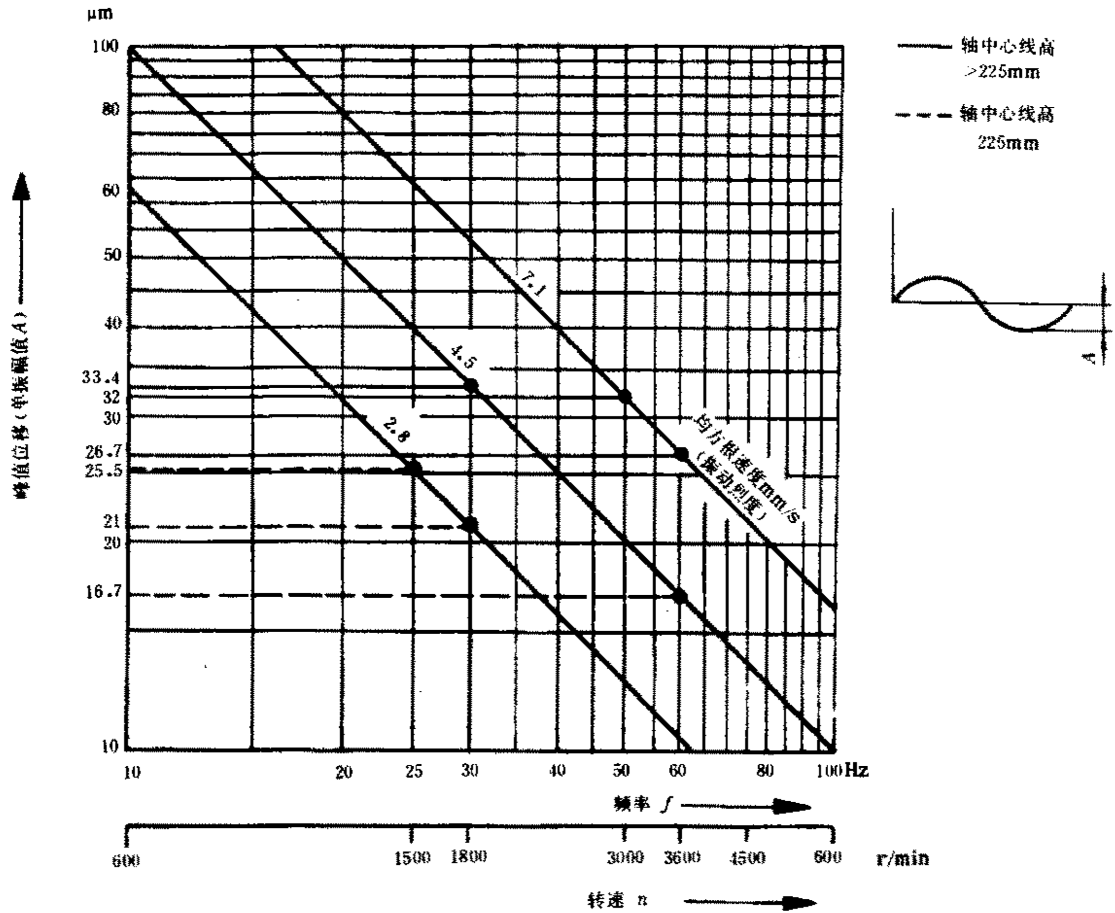
图 B1 不同的均方根速度值时单振幅值 A 与转速的函数关系 (均方根 r. m. s 的定义见 GB 6075)
