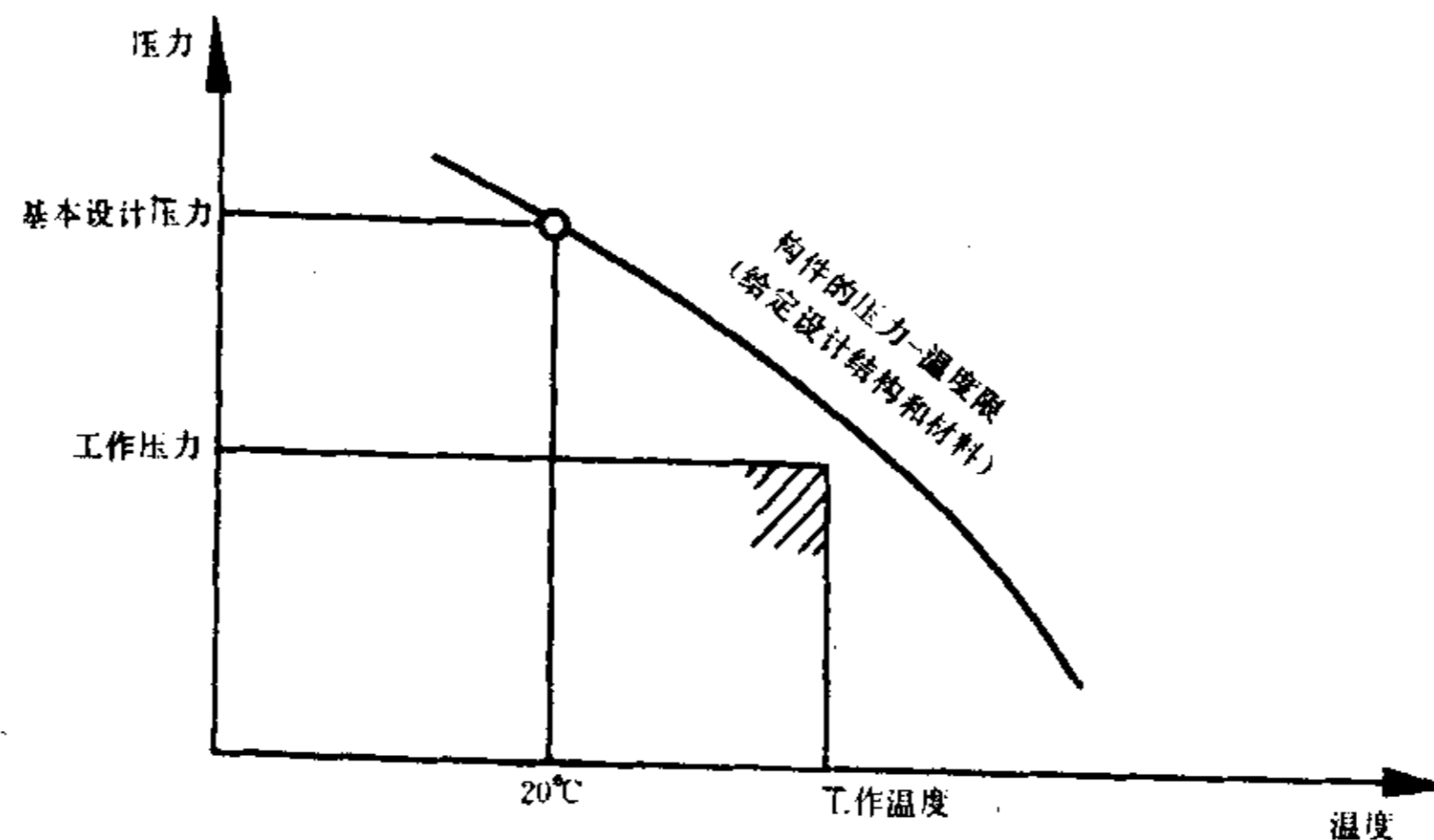
图 1 压力-温度特性
