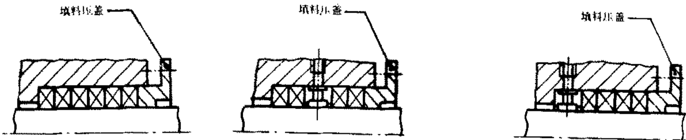
P2 有填料环(用于密封、 阻隔、冷却等液体的注 入或循环)的软填料
