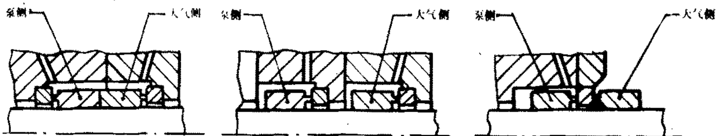
D1 背靠背配置
